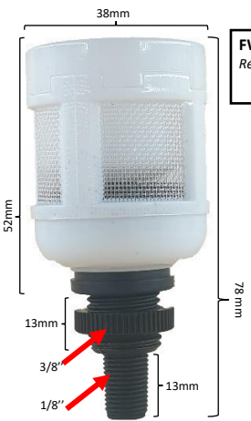
NGF 02-12 Référence : 4DEPFS129025 Pour marque DELTECH
