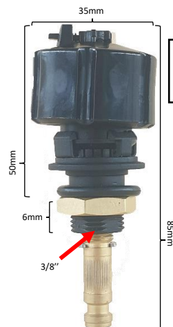
G 17 Référence : 4PNGADPURG17 Pour marque ATLAS COPCO
