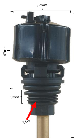
G 20 Référence : 4PNGADPURG20 Pour marque ZANDER / OMI / KAESER / BEKO / HANKISON / DONALDSON DF
