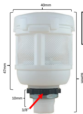
TYPE II Référence : 4DEPFS6051400 Pour marque COMPAIR / NORGREN / MIKROPOR
