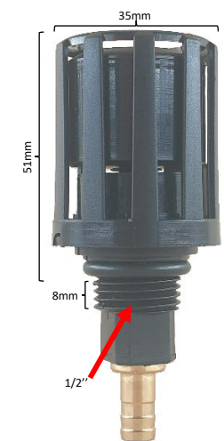
PSL 15 Référence : 4OAFIS000016 Pour marque ABAC / ATLAS COPCO / CREYSSENSAC
