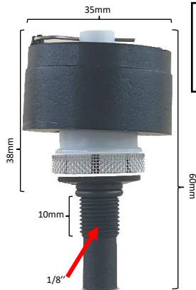
WAD Référence : 4DEPFS061095 Pour marque WATTS / ULTRAFILTER 80 / COMPAIR 80
