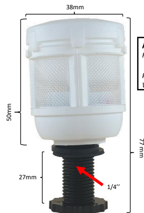
TYPE II Référence : 4DEPFS6051400 Pour marque COMPAIR / NORGREN / MIKROPOR
